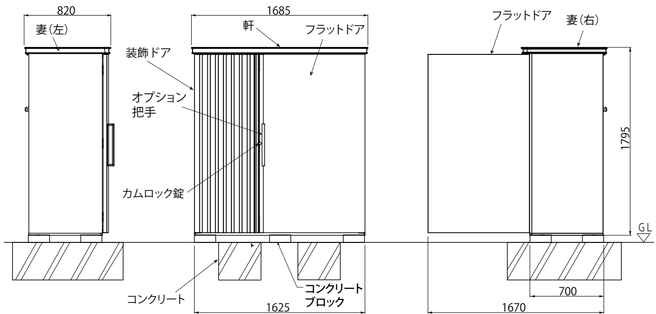
左側面図
